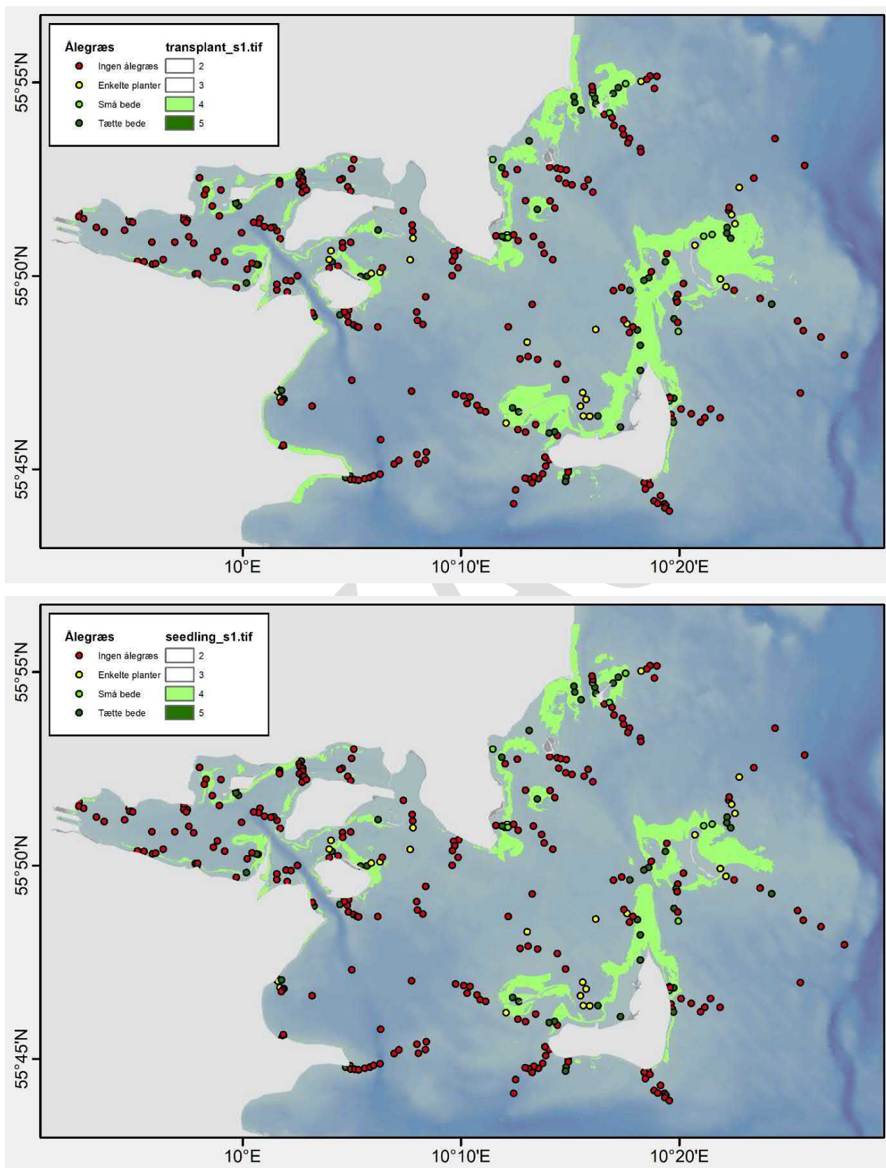
Figur 7-5 Ålegræsmodelresultater af to model-output: transplant (øverst) og seedling (nederst). Punkter repræsenterer observerede data fra DTU Aquas undersøgelser i 2016, mens lysegrønne områder repræsenterer modellens output for "gode" forhold for ålegræssets forekomst.
