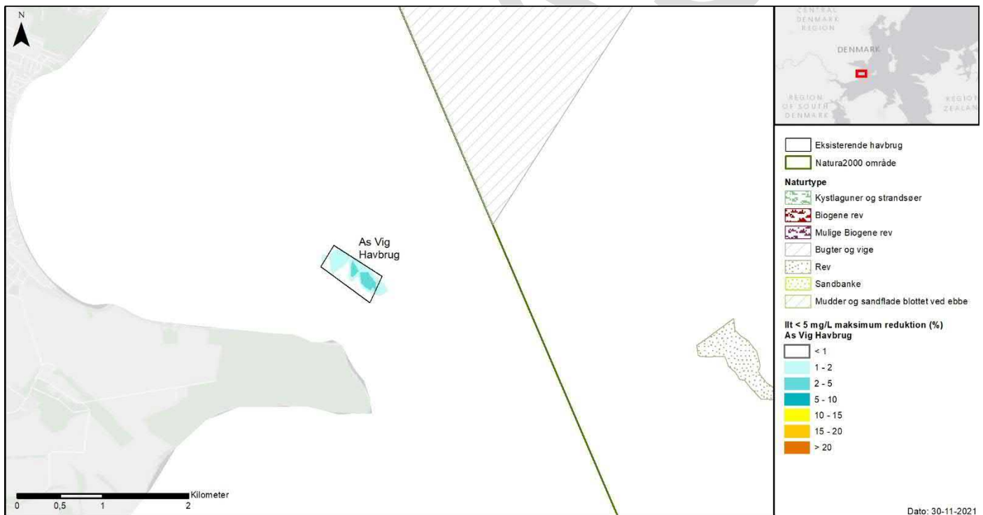
Figur 8-10 Maksimal procentvise ændring i gennemsnitlig daglig iltkoncentration ved bunden (i 5-års perioden) ved iltkoncentration < 5 mg L -1 for As Vig Havbrug. Ændringer > 10% angiver grænsen for påvirkning foranlediget af ændring i bundvandets koncentration af ilt. Øverst: oversigtskort med hele Natura 2000-området 56. Nederst: zoom på området omkring As Vig Havbrug.
