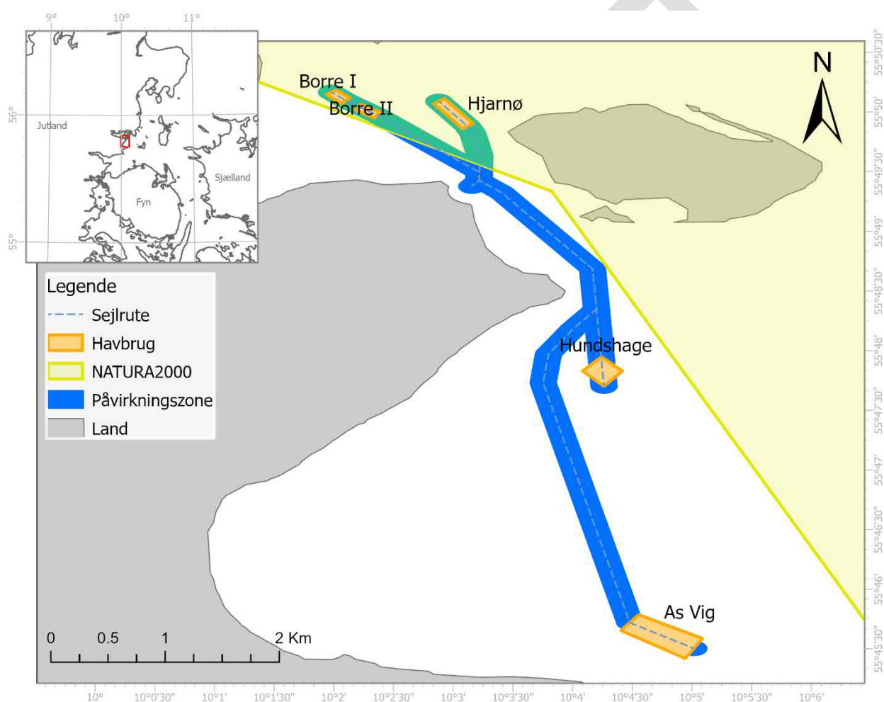
Figur 8-42 Påvirkningszoner for As Vig, Borre I, Borre II, Hjarnø og Hundshage Havbrug. Stiplet linje angiver sejlruterne fra Snaptun Havn og til havbrugene. Den blå polygon angiver den effektive påvirkningszone (2*120 m), som er grøn ved overlap med N56.
