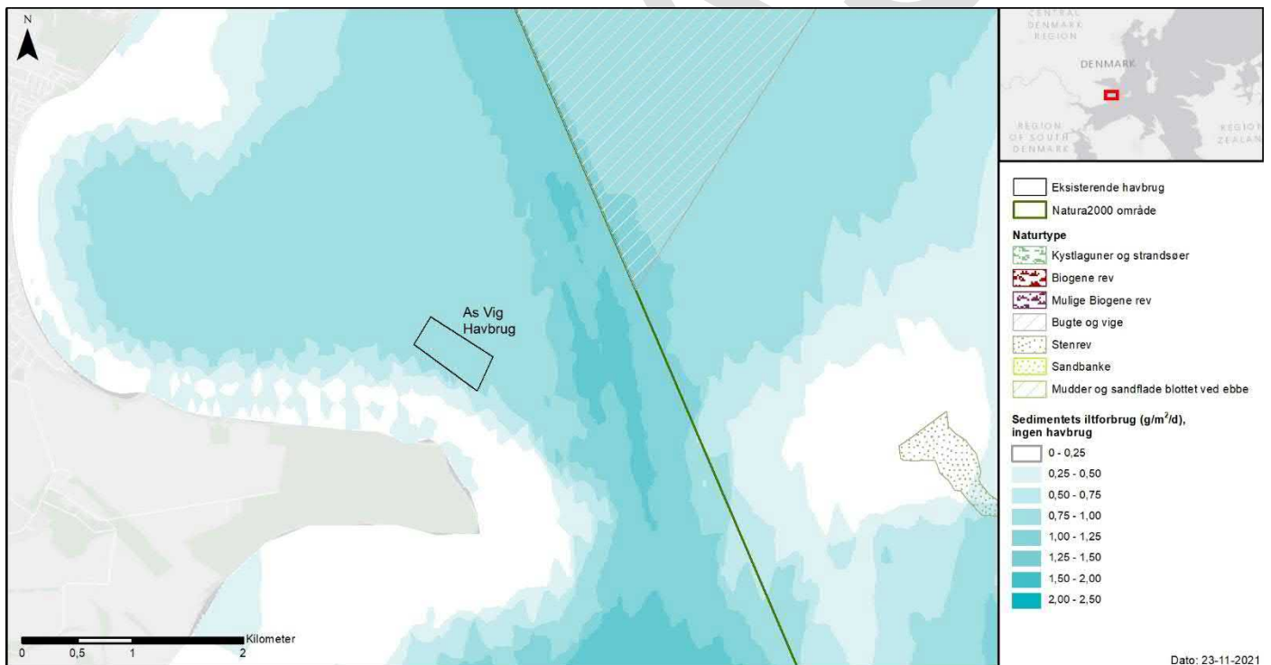
Figur 8-1 Oversigt over sedimentets årgennemsnitlige iltforbrug (g O 2 m -2 dag -1 ) i perioden 2014-2018. Øverst: oversigtskort med hele Natura 2000-område 56. Nederst: zoom på området omkring As Vig Havbrug.
