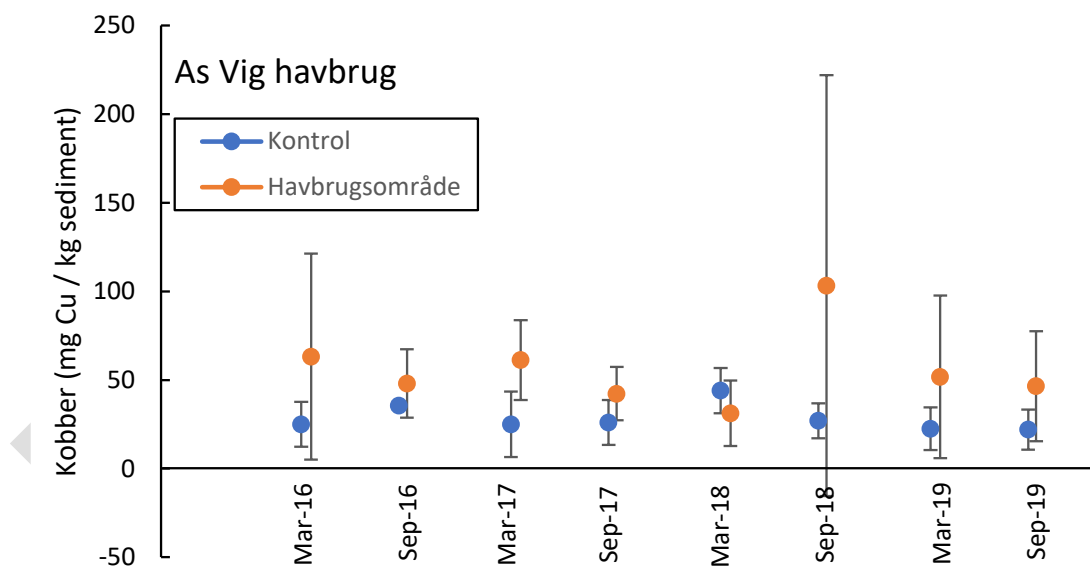
Figur 8-46 Tidlig variation i koncentrationen af kobber i kontrolområde og havbrugsområde (inkluderende sedimentprøver indsamlet under opdrætsringene) for As Vig Havbrug. Middelverdier og \pm standardafvigelse vist.
