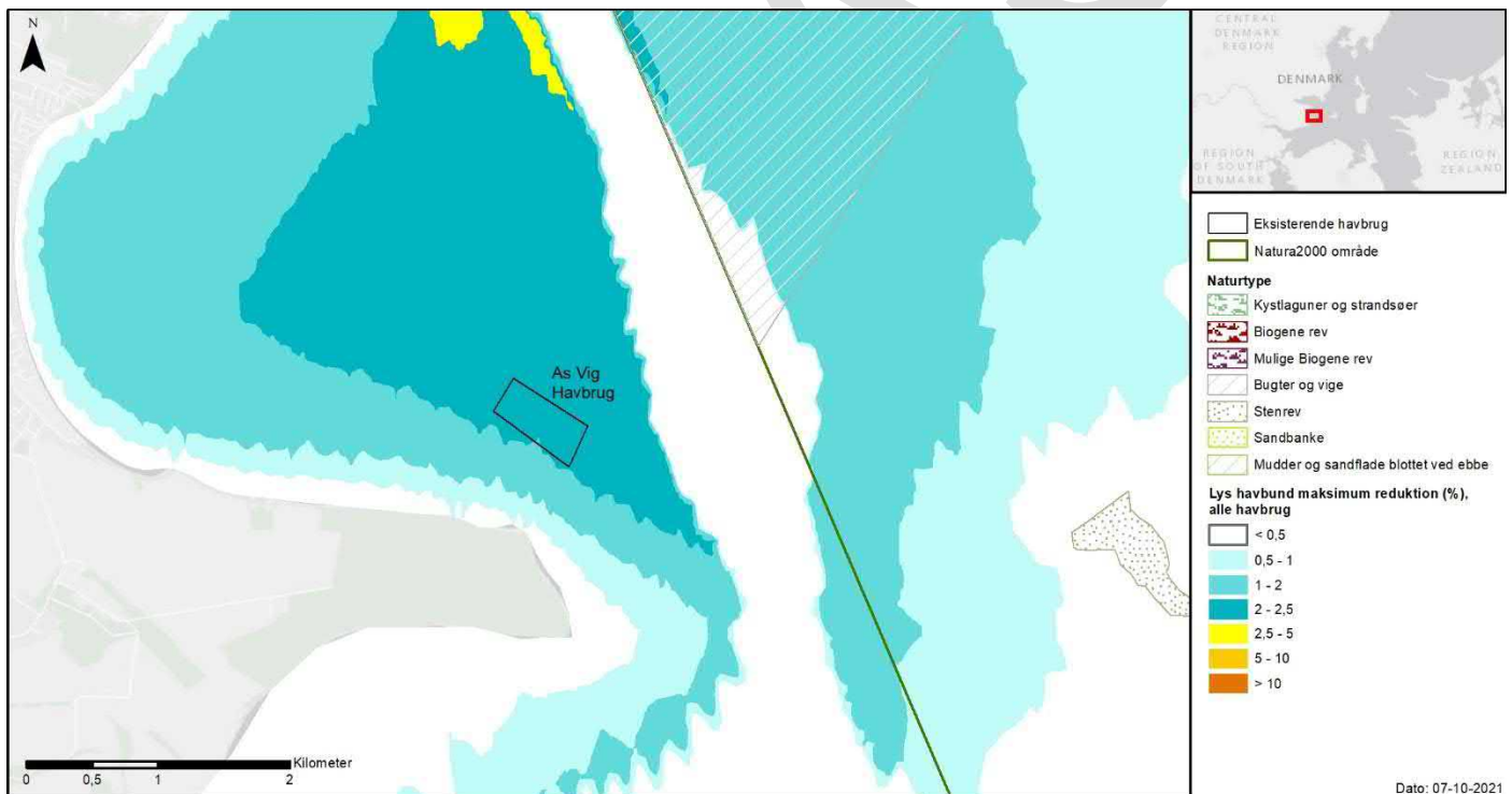
Figur 8-18 Maksimal procentvis ændring i lys ved bunden (for produktionsperioden) i lysintervallet 17,5 - 300 \mu\text{E m}^{-2} \text{s}^{-1} , As Vig Havbrug kumuleret med omkringliggende havbrug. Ændringer > 2,5% angiver grænsen for påvirkning foranlediget af ændring i lys ved bunden. Øverst: oversigtskort med hele Natura 2000-område 56. Nederst: zoom på området omkring As Vig Havbrug.
