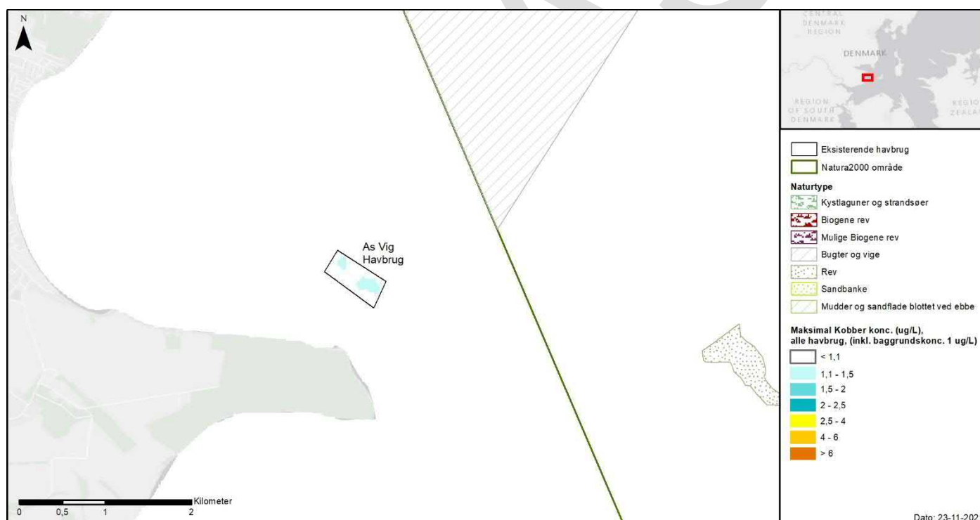
Figur 8-30 Maksimumkoncentrationer af tilført kobber i overfladen (0-5 m) som følge af samtidig anvendelse ved alle 5 havbrug i juni-august. Øverst: oversigtskort med hele Natura 2000-område 56. Nederst: zoom på området omkring As Vig Havbrug.
